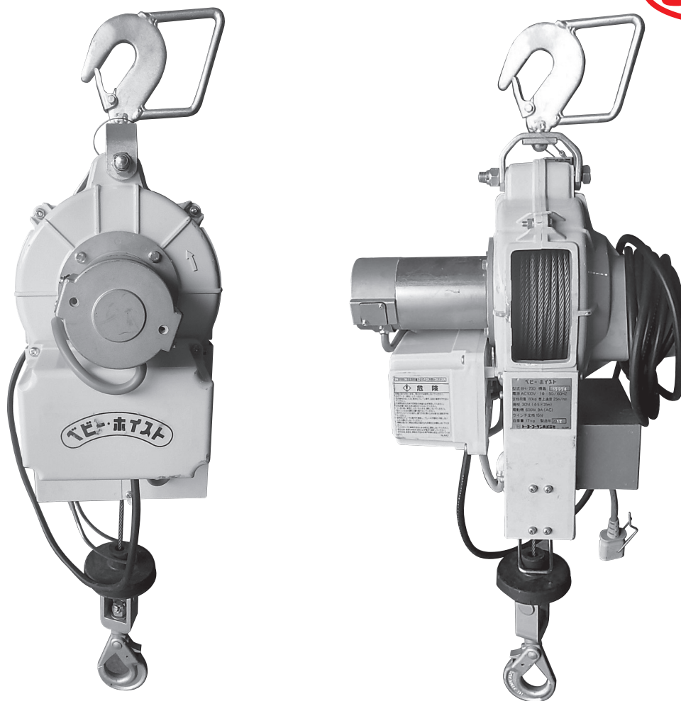
100Vベビーホイスト トーヨーコーケンBHシリーズ
