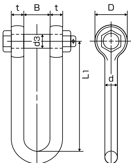
■ 強力長シャックル 寸法図
